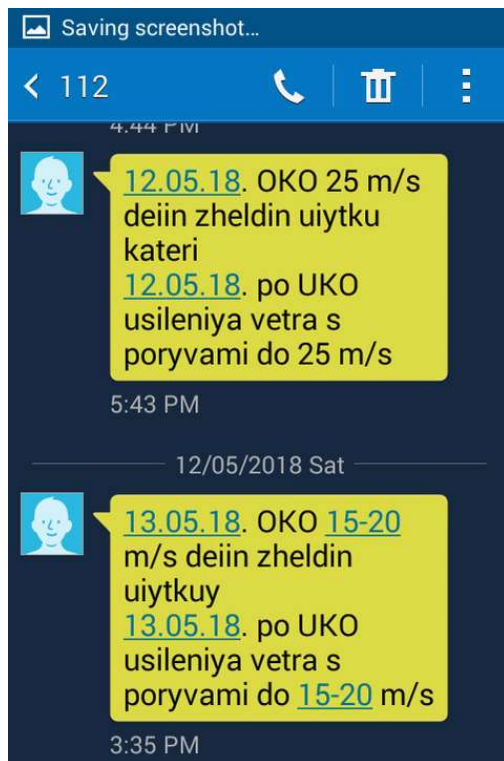
również 12 maja, wiatr 15-20 m/s. 13 to samo plus burza.
