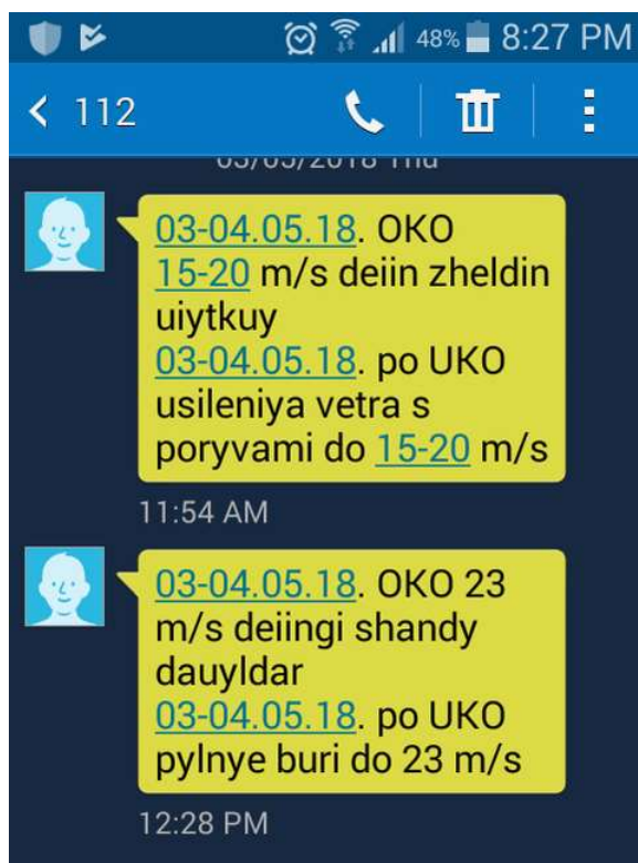
3-4 maja, wiatry niosące pył, 15-20 m/s
